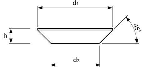
Geometrie Senkkopf bei Ausführung SZ-SK.
